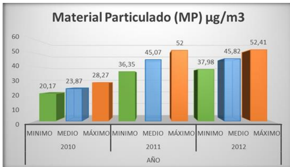
Gráfico 3 Material particulado Cajicá
