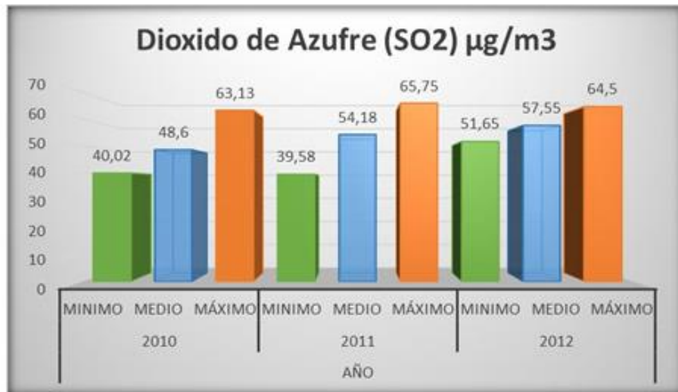
Gráfico 1 Dióxido de Azufre Cajicá
