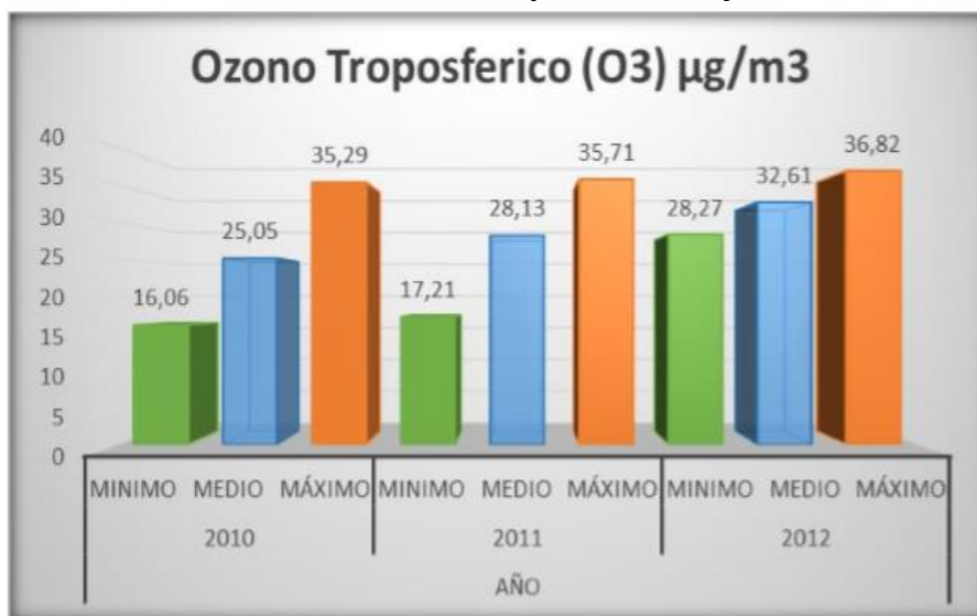
Gráfico 5 Ozono Troposférico Cajicá
