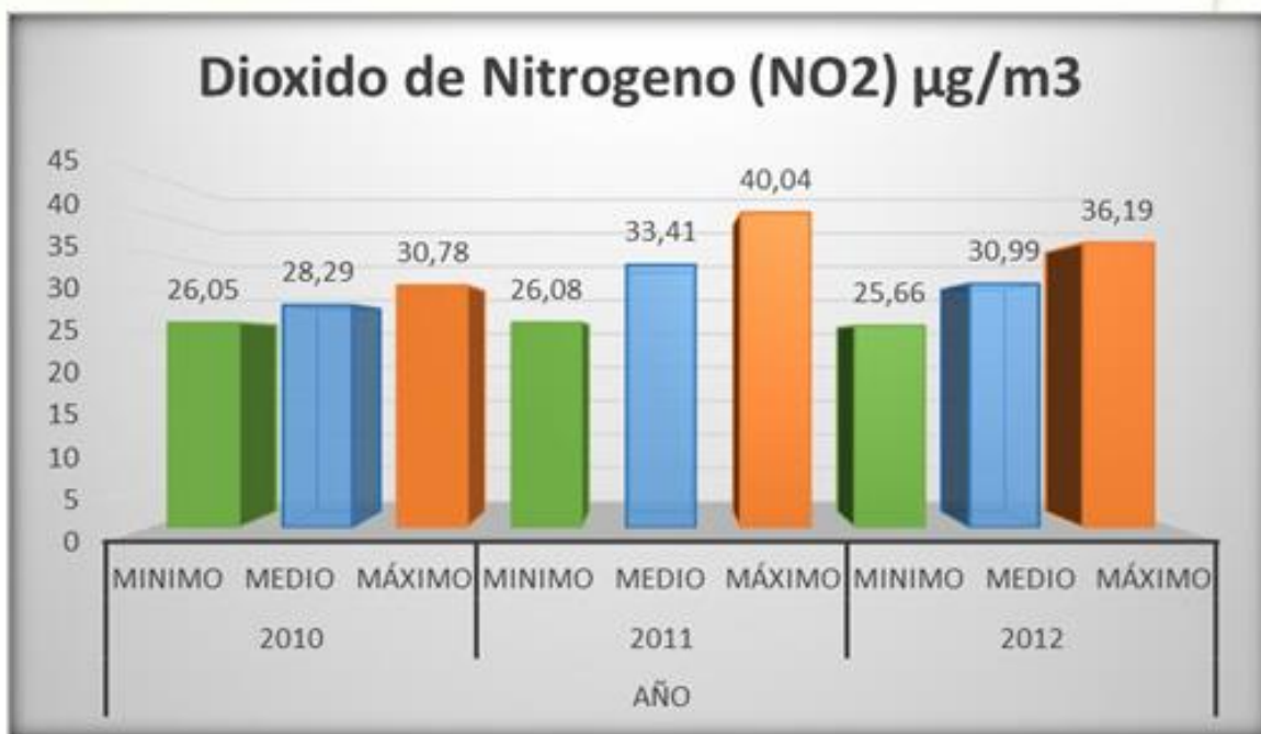
Gráfico 2 Dióxido de Nitrógeno Cajicá
