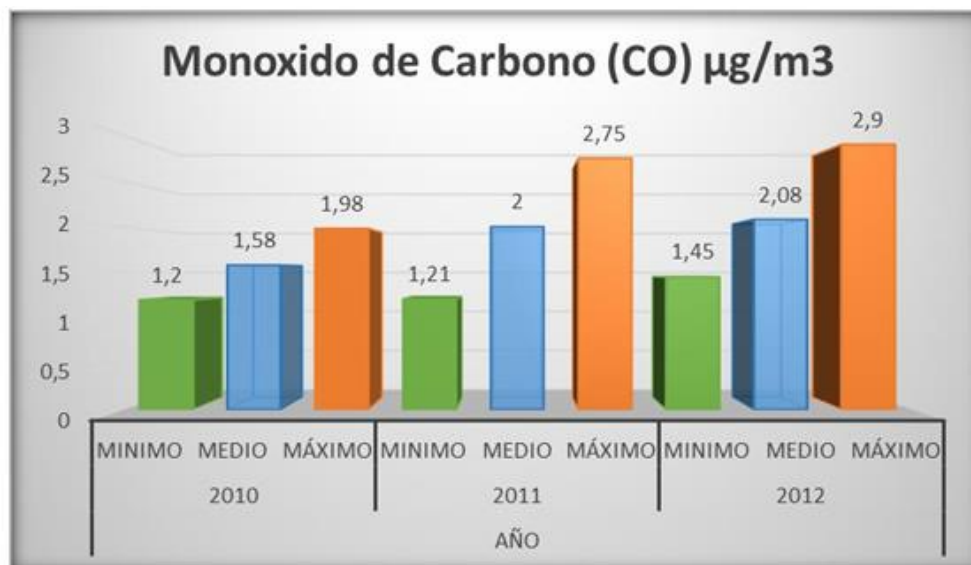
Gráfico 4 Monóxido de carbono Cajicá
